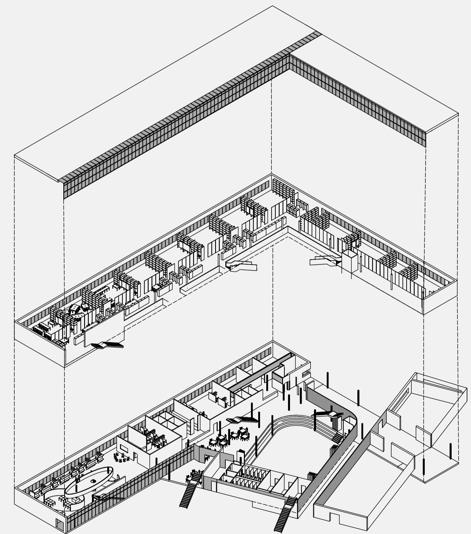
explosionszeichnung eg+og
