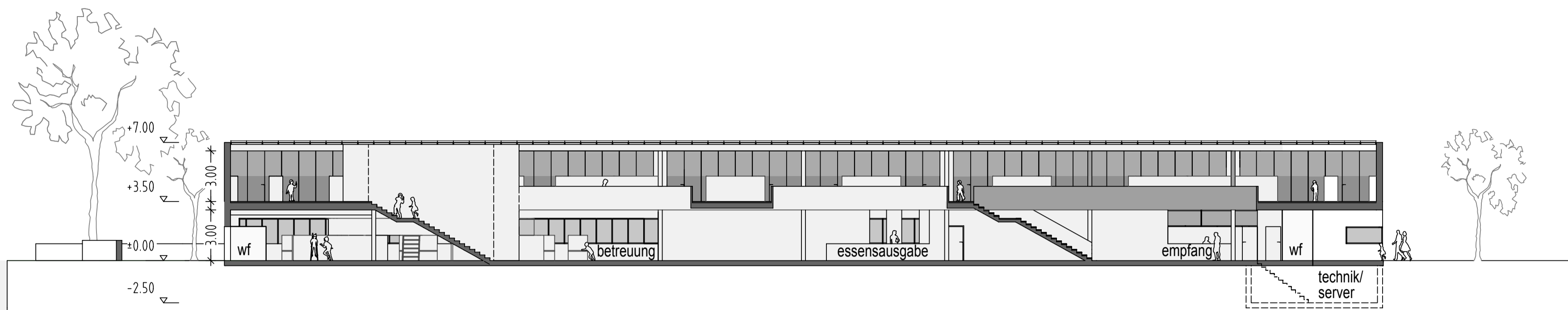
schnitt A-A
