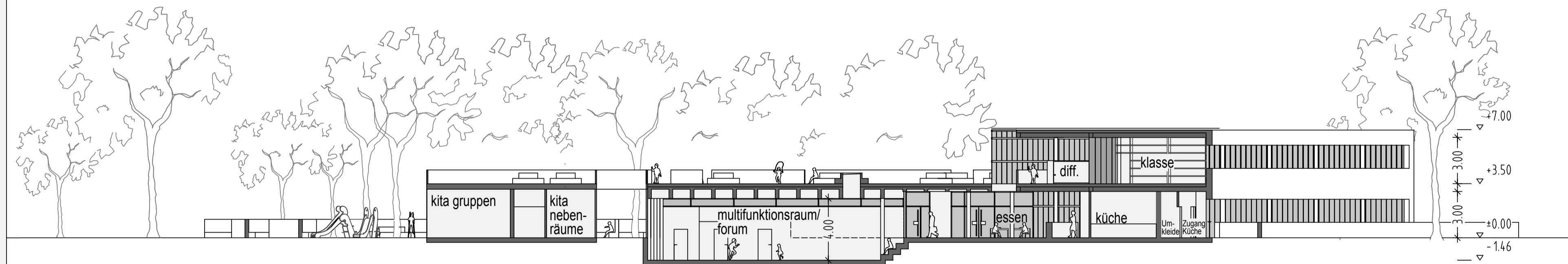
schnitt C-C
