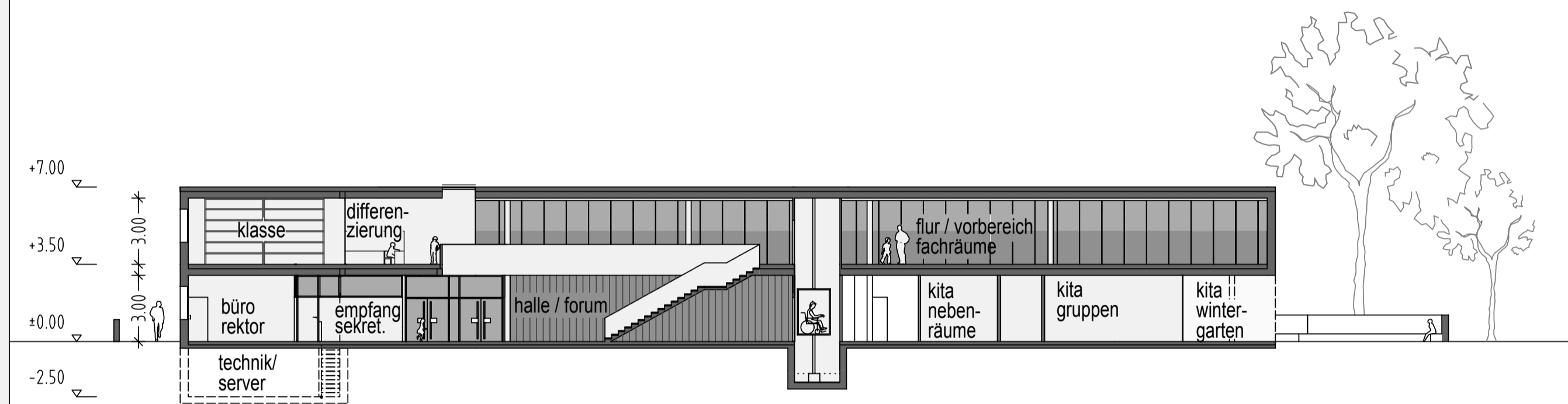
schnitt B-B
