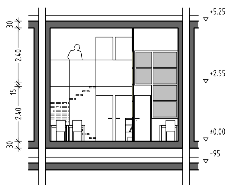
sección B1-B1 e 1/100
